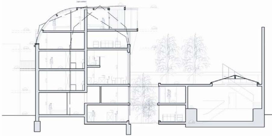
coupe b-b
